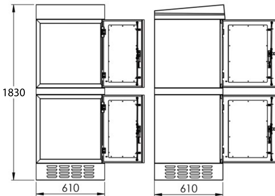
WIDOK PRZODU
